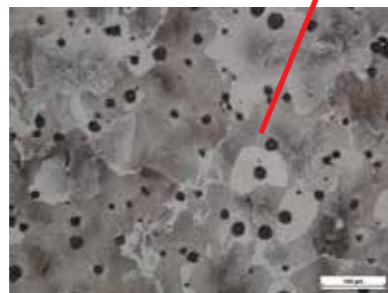
Perlito-Bainitique
